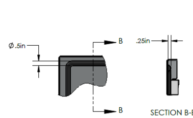
DOOR GASKET
